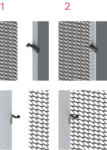
Detalles de fijación
